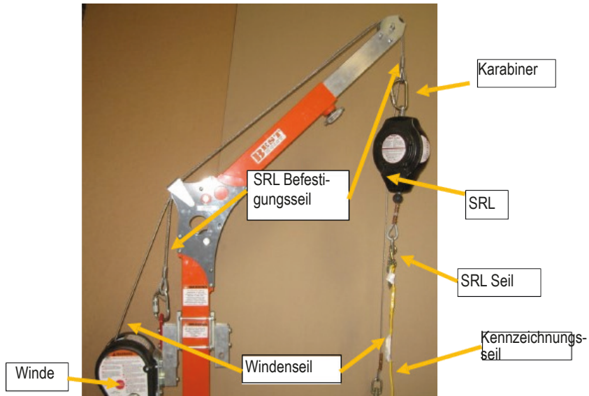
Abbildung 10 Optionale SRL Montage/Anschlagseil Installation
