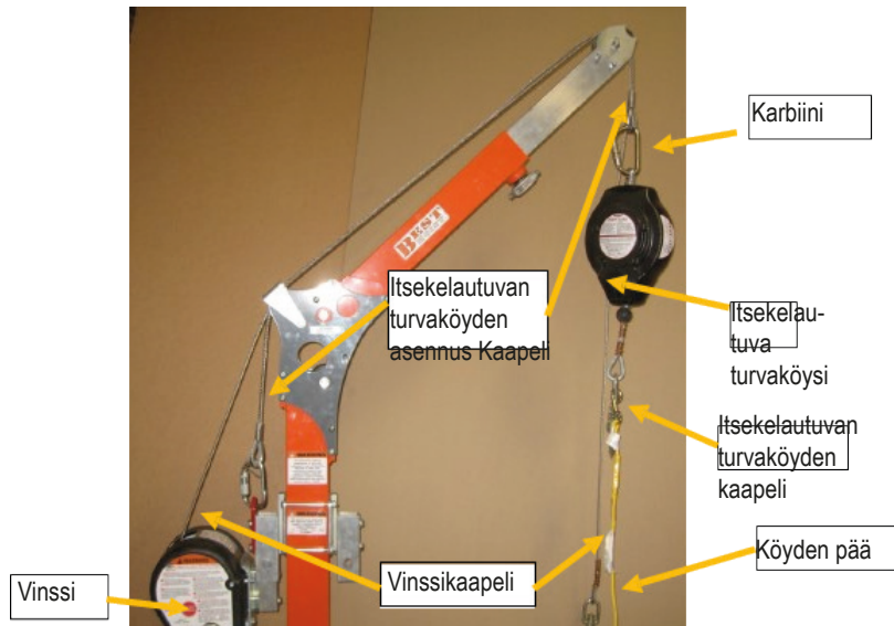
Kuva 10, Valinnaisen itsekelaavan turvaköyden asennusankkurikaapelin asennus
