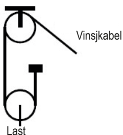
Figur 3, Typisk to-dels enkelttrukket system
