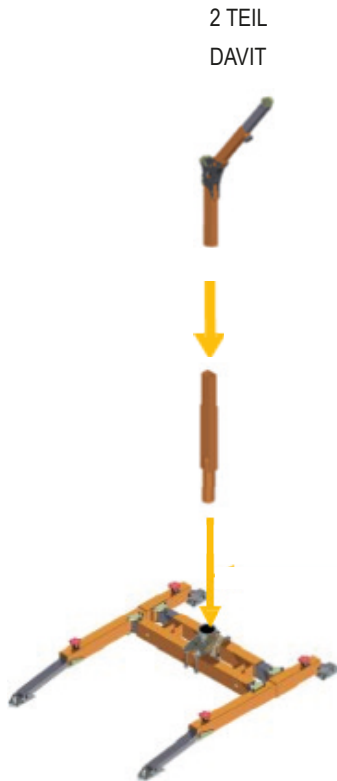
Abbildung 8, Installation des JACKPOD Davit LM Arm bis JACKPOD Base Portable
