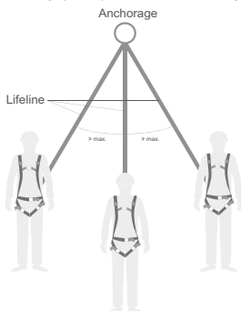
Abbildung 5 Maximaler Schwenkwinkel
