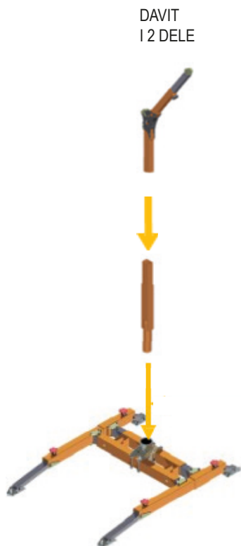
Figur 8, montering af Jackpod Davit LM Arm til monteringssokkel i Jackpod Base Portable
