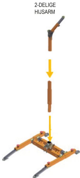
Afbeelding 8, installatie van het bodemframe van de hijsarm Jackpod Davit LM tot Jackpod Base Portable
