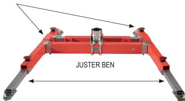
Figur 6, Montering og justering av Portable base
