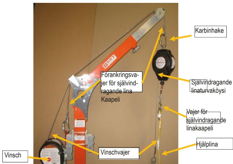
Bild 10 - Installation av förankringsvajer för självindragande lin (tillval)
