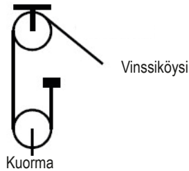
Kuva 3, Tyypillinen 2-osainen yksinkertaisesti pujotettu järjestelmä
