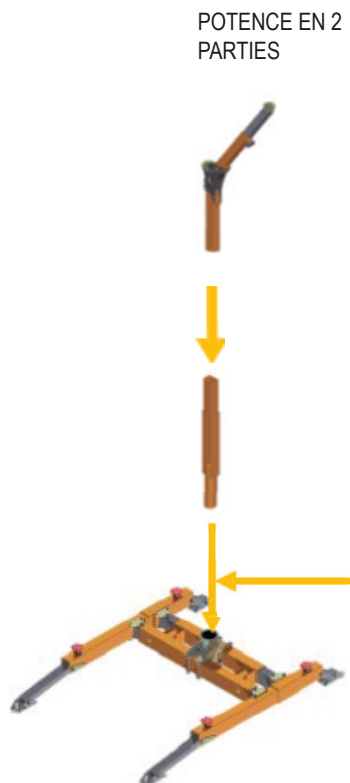
Illustration 8, installation du bras de potence Jackpod Davit LM sur Jackpod Base Portable
