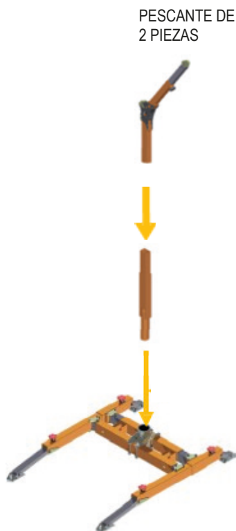
Figura 8, Instalación del brazo del pescante Jackpod Davit LM en Jackpod Base Portable
