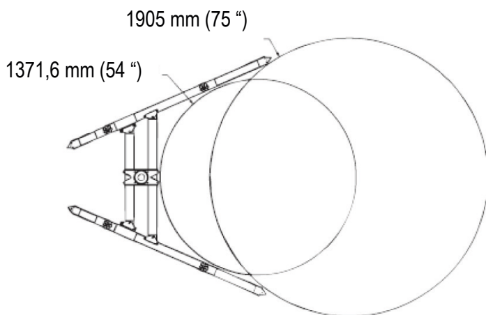
Abbildung 7 Bandbreite an Öffnungsgrößen für den JACKPOD Base Portable
