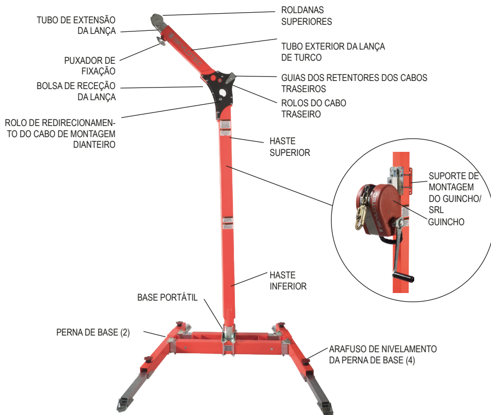
Figura 1, Peças e localização do Sistema de turco da Série
