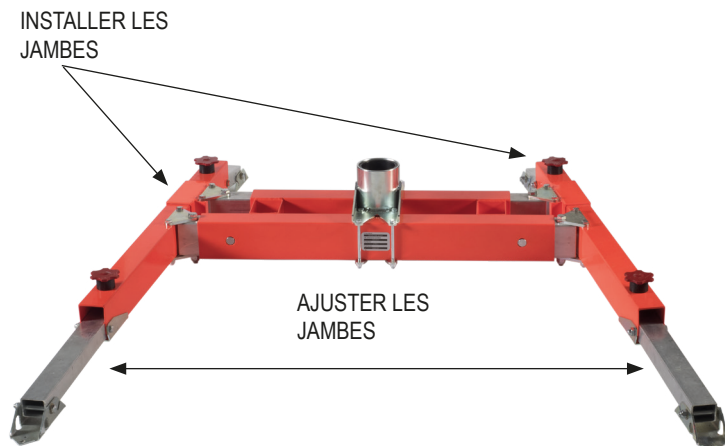
Illustration 6, assemblage et ajustage de Jackpod Base Portable
