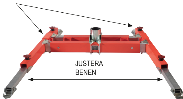
Bild 6 - Installation och justering av Jackpod Base Portable
