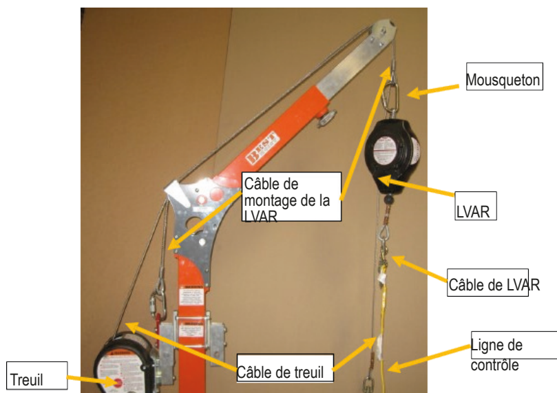
Illustration 10, Installation du câble d'ancrage en option pour le montage d'une LVAR
