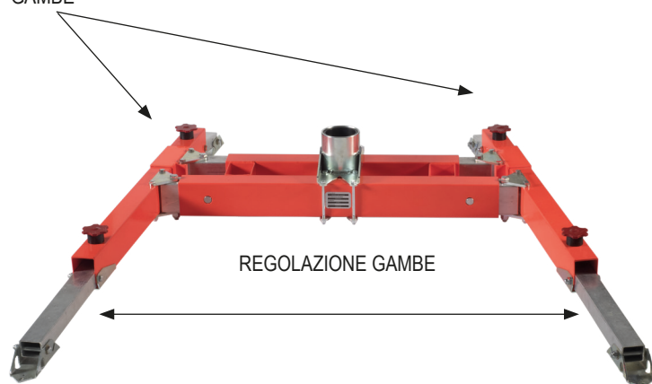
Figura 6, Assemblaggio e regolazione della base portatile
