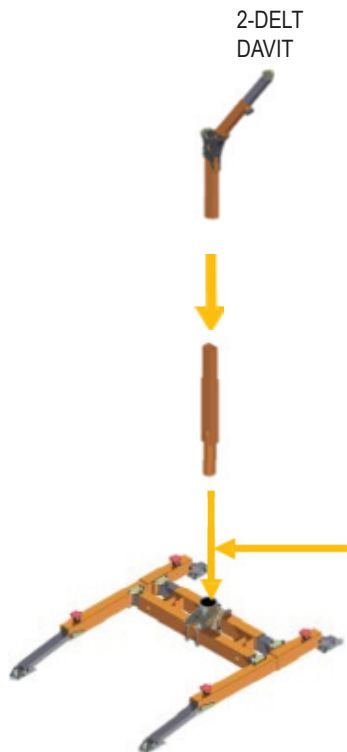
Figur 8, Installasjon av Jackpod Davit LM Arm til Jackpod Base Portable
